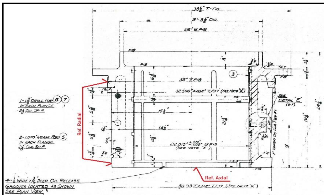
Figura 1 - Referências para centragem e usinagem do mancal (Desenho 53585)
