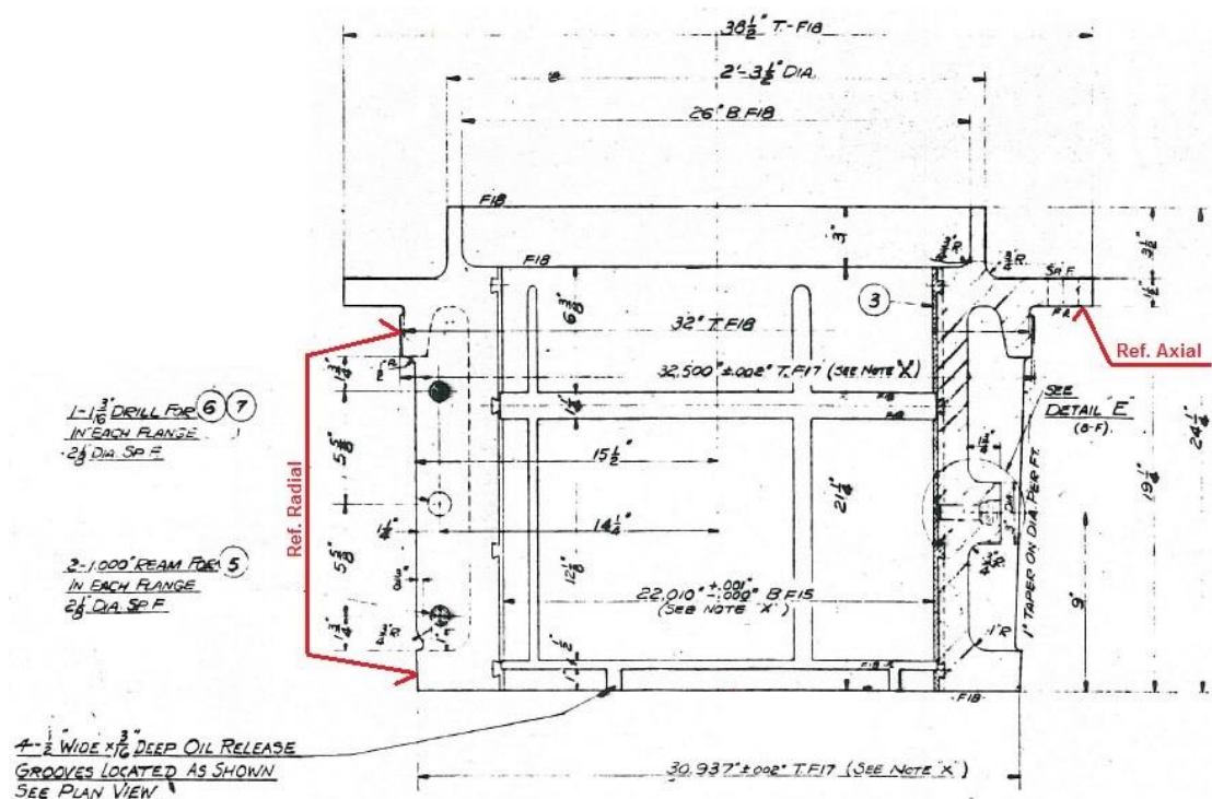
Figura 1 - Referências para centragem e usinagem do mancal (Desenho 53585)
